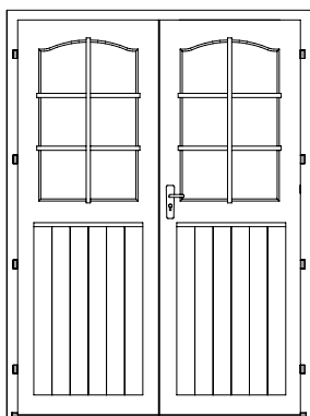
Doppeltür 70 mm ISO 1425 x 1955 mm 1 st.
