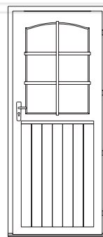
19 ISO 70 mm 840 x 1955 mm 1x
