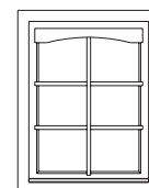
21 ISO 70 mm 765 x 990 mm 1x
