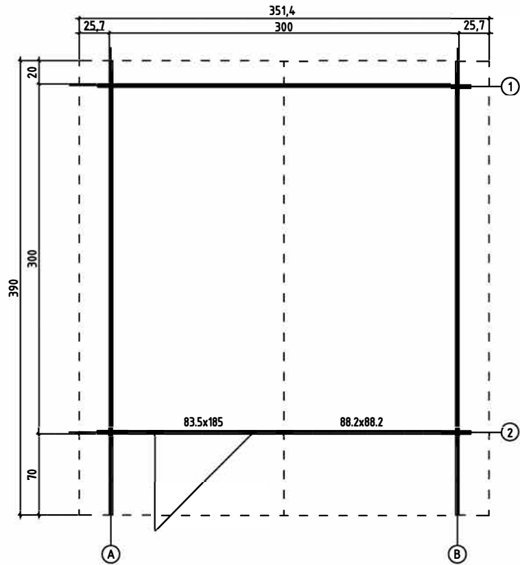
GROUNDPLAN - GRUNDPLAN - PLAN DE MASSE
